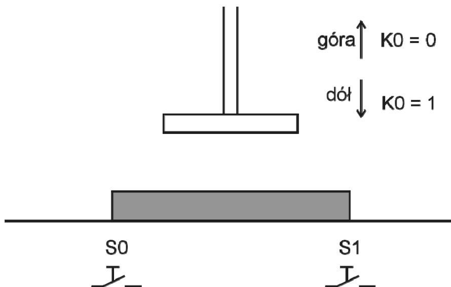
Rys. 1. Schemat technologiczny prasy
